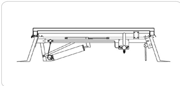
Dunkelklappe MISTRAL
